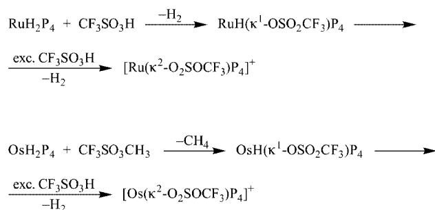
Scheme 2. P = P(OEt) 3 , PPh(OEt) 2
